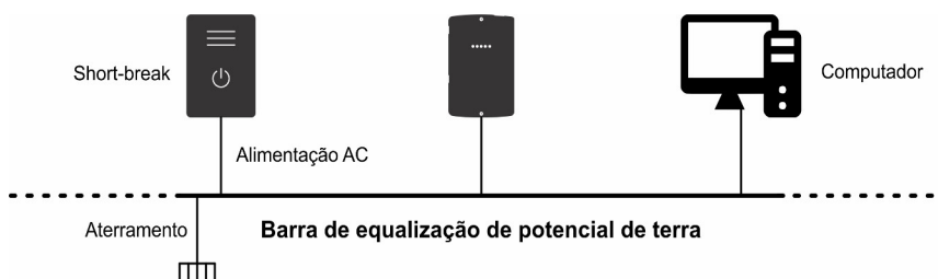
Figura 9: Aterramento
