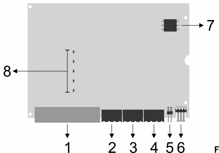
Figura 2: Placa Cpu
