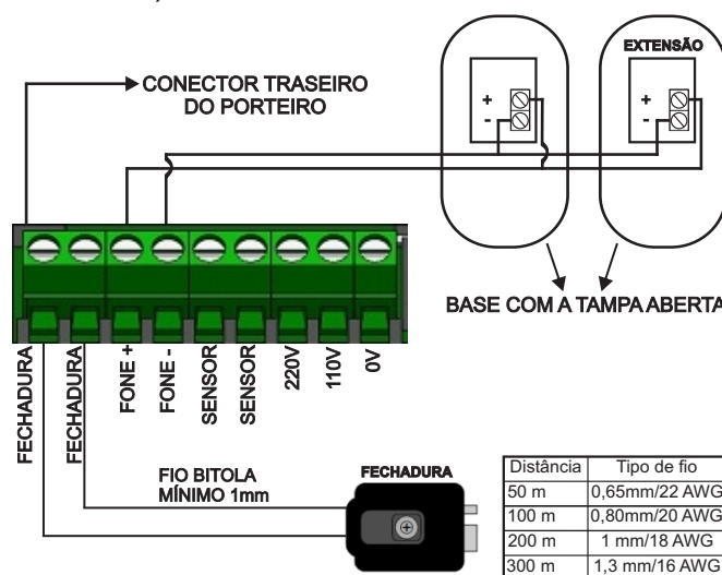
Figura 1: Instalação
